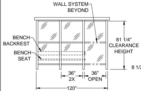
ELEVATION A
